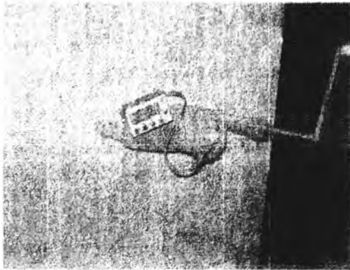
Рис. 1 Определение прочности бетона методом отрыва со скалыванием.
